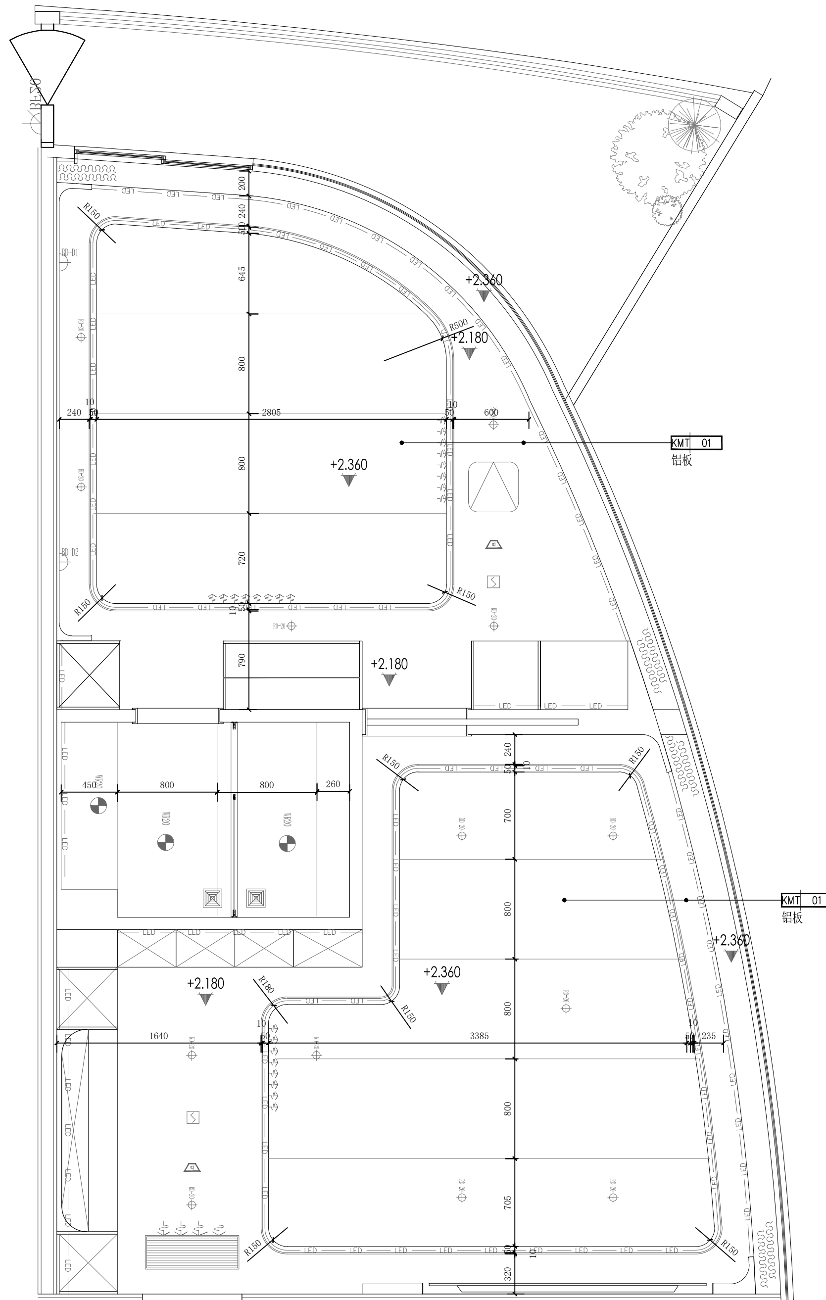
豪华套房天花布置图
