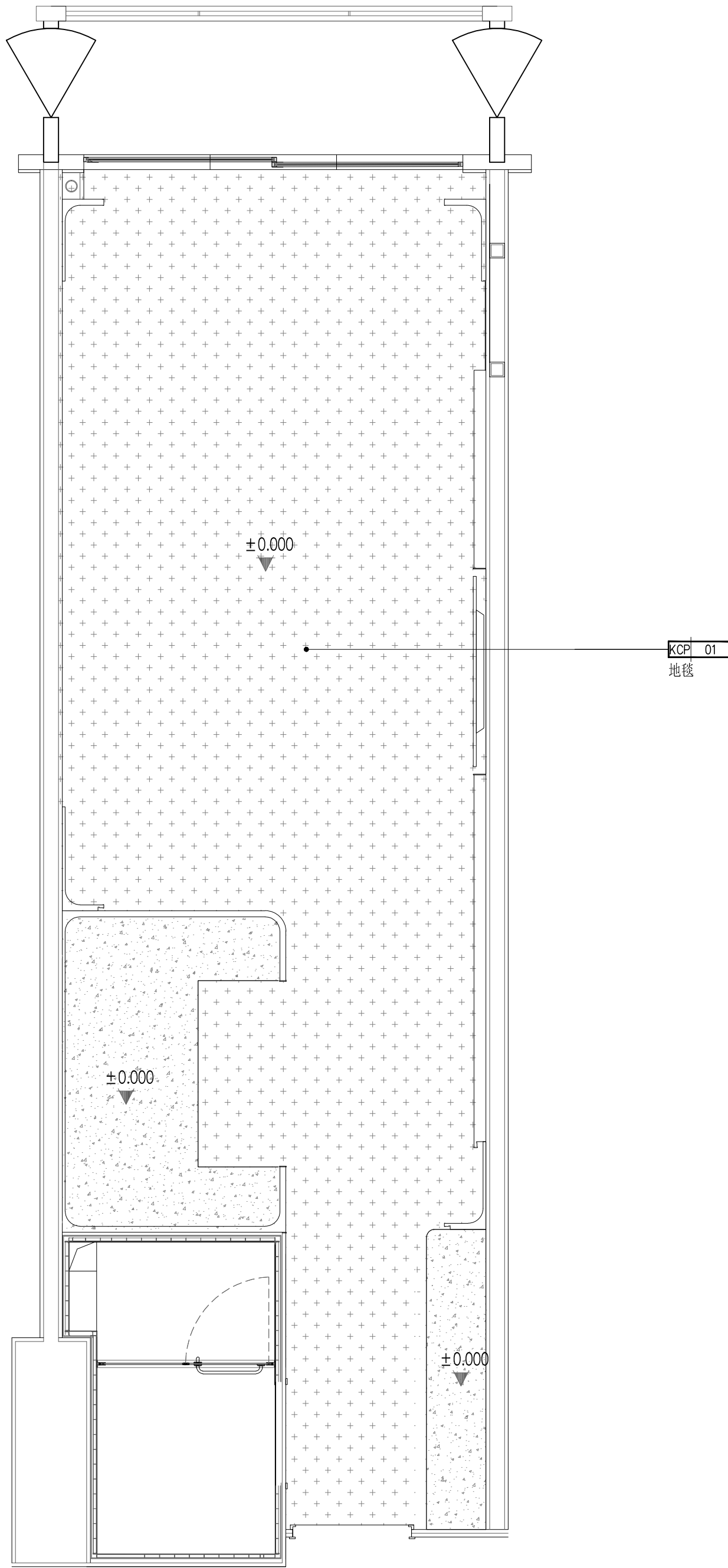
亲子套房地面铺装图 1:30@A2
