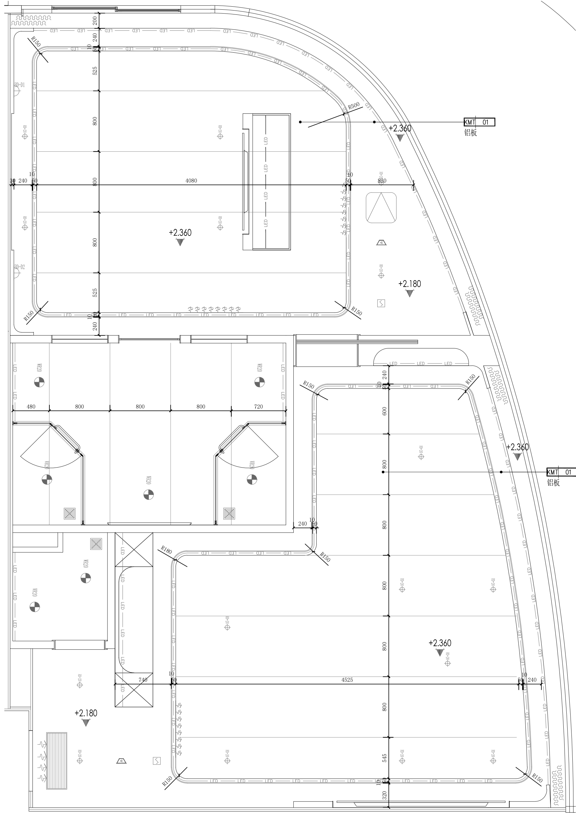
总统套房天花布置图 1:30@A2
