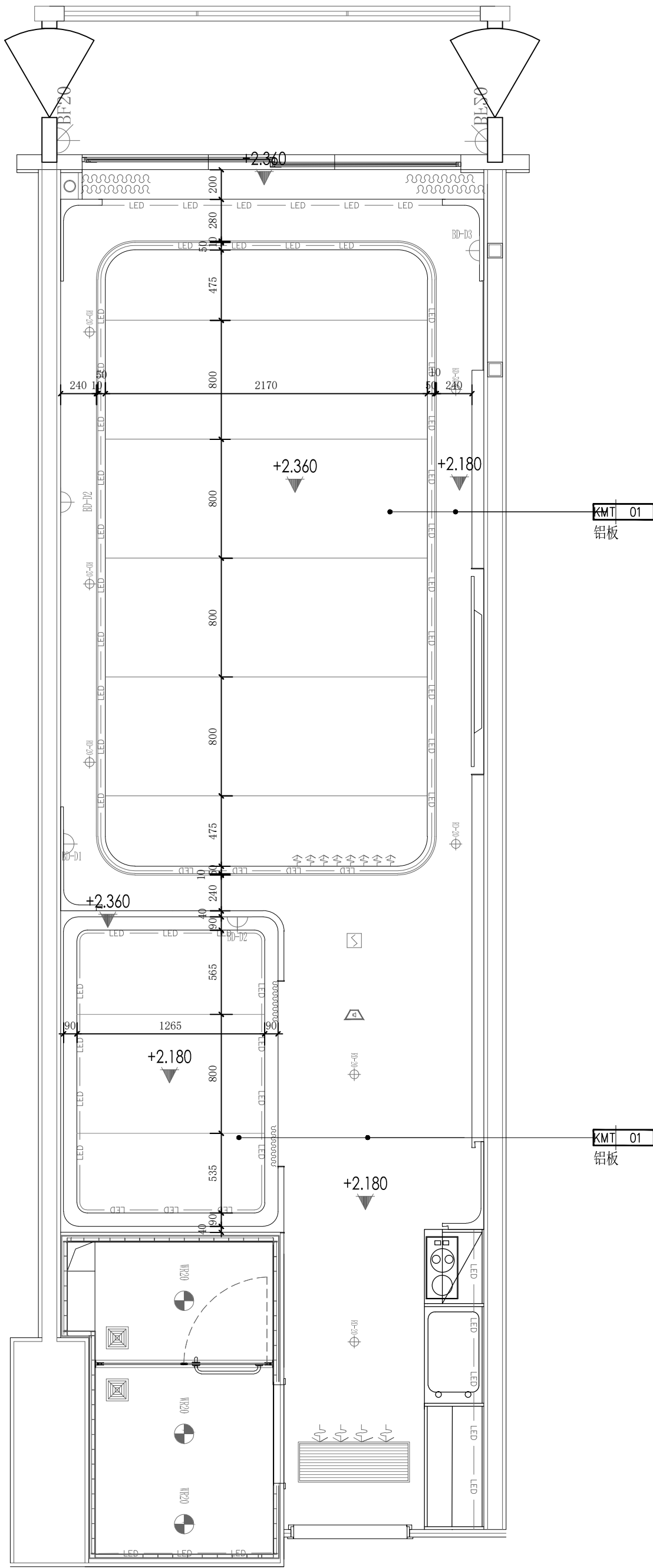
亲子套房天花布置图 1:30@A2
